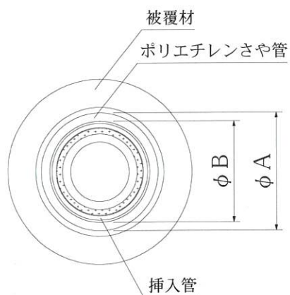
挿入管③
