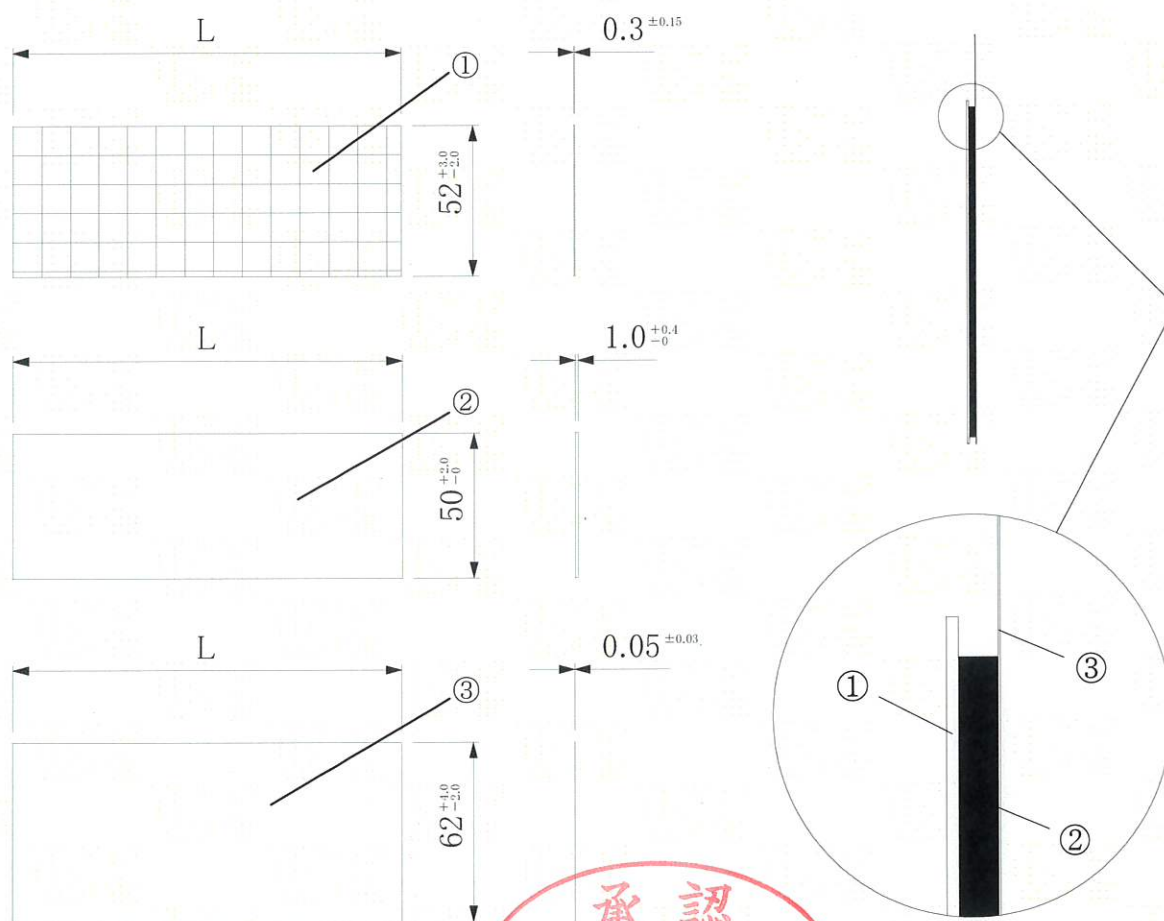
図-2 IRG-Tの断面図
