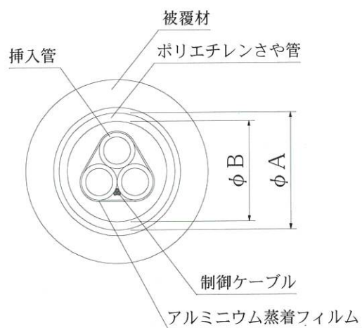
挿入管④、⑤
