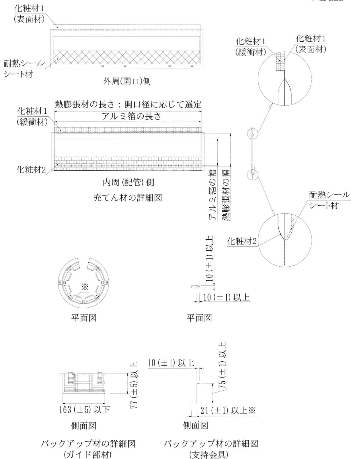
図3 構造説明図
