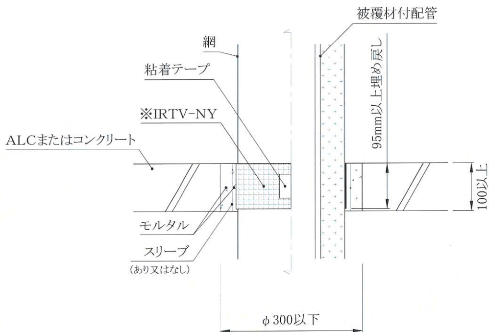
断面図
