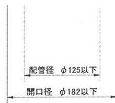
断面図
