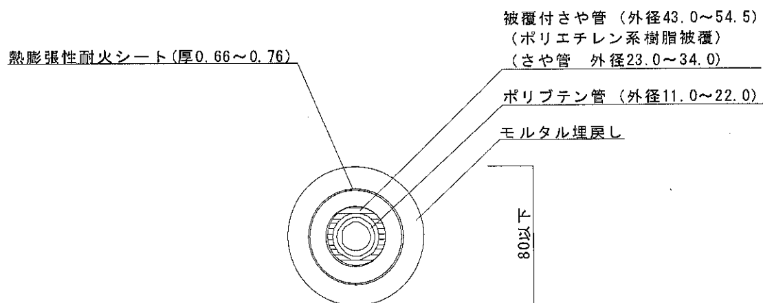
<正面図>
