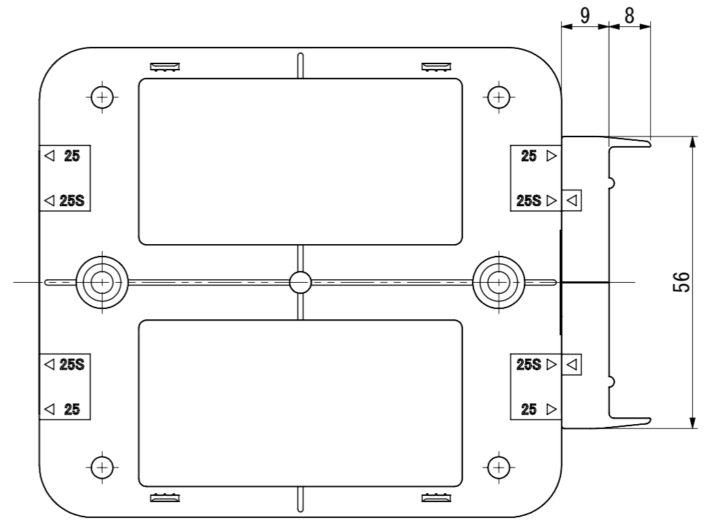
JEC-25S使用時
