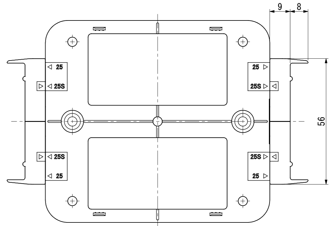
JTC-25S使用時
