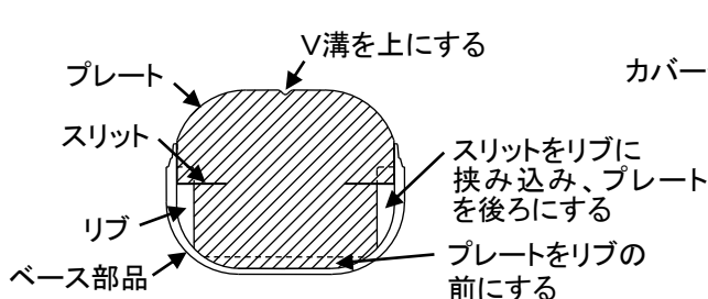
【図1: 取り付け方法】
