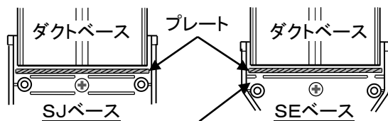
【図3: 差し込み位置】
