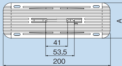
寸法図
